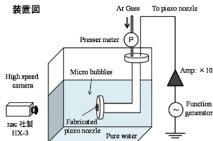
圧電振動ノズル
