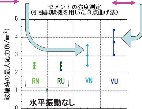
図5: 超音波照射によるモルタルの破壊強度の増加実験
